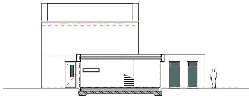
- doorsnede B-B -
