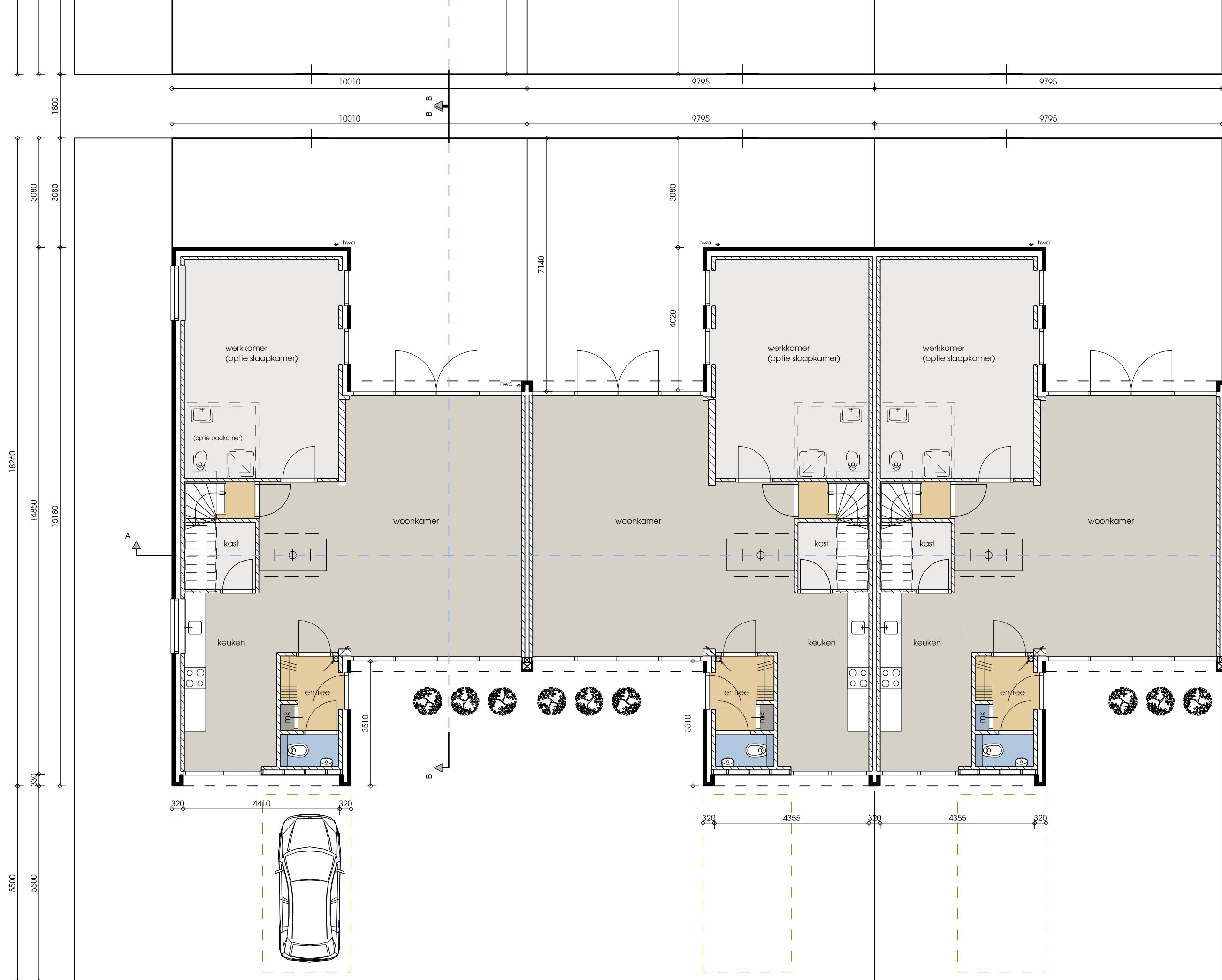
- begane grond -
